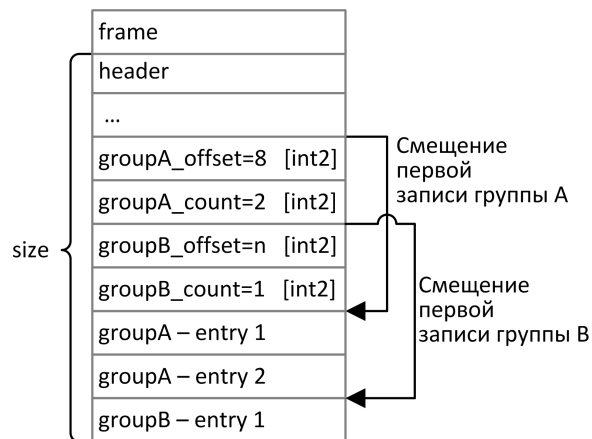
Рисунок 2.1. Схема сообщения с двумя повторяющимися компонентами
