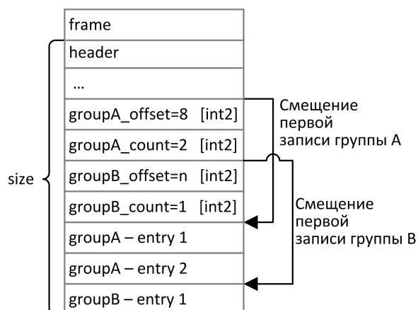
Рисунок 3.1. Схема сообщения с двумя повторяющимися компонентами
